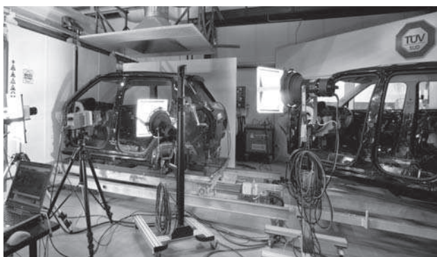
Celkový pohled na pracoviště zkoušek airbagů ve zkušebně TÜV SÜD Czech v Mladé Boleslavi.
